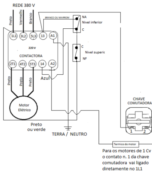
Figura 01 – Ligação dos bornes
